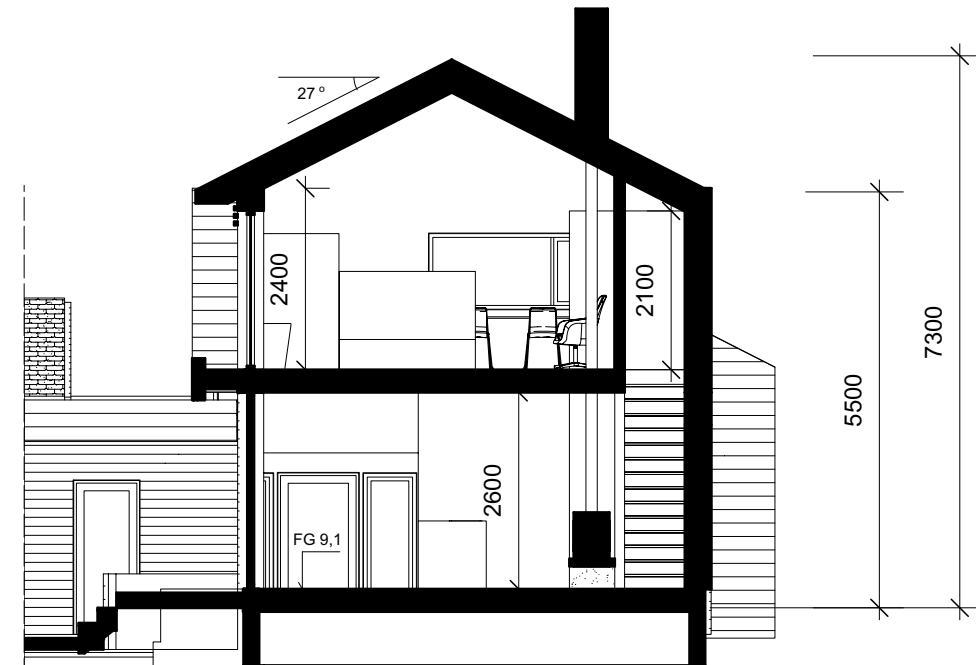
Snitt C-C
