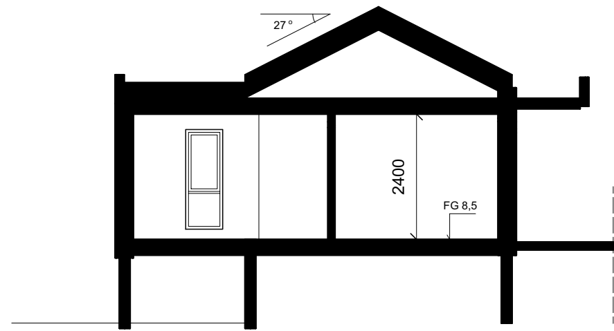
Snitt B-B
