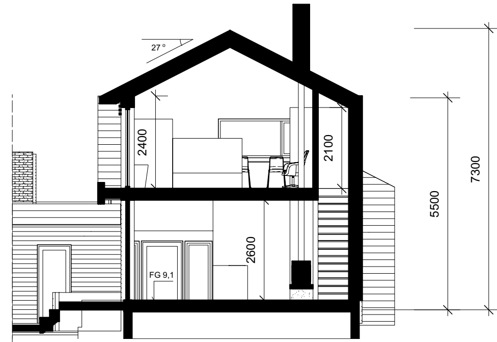
Snitt C-C
