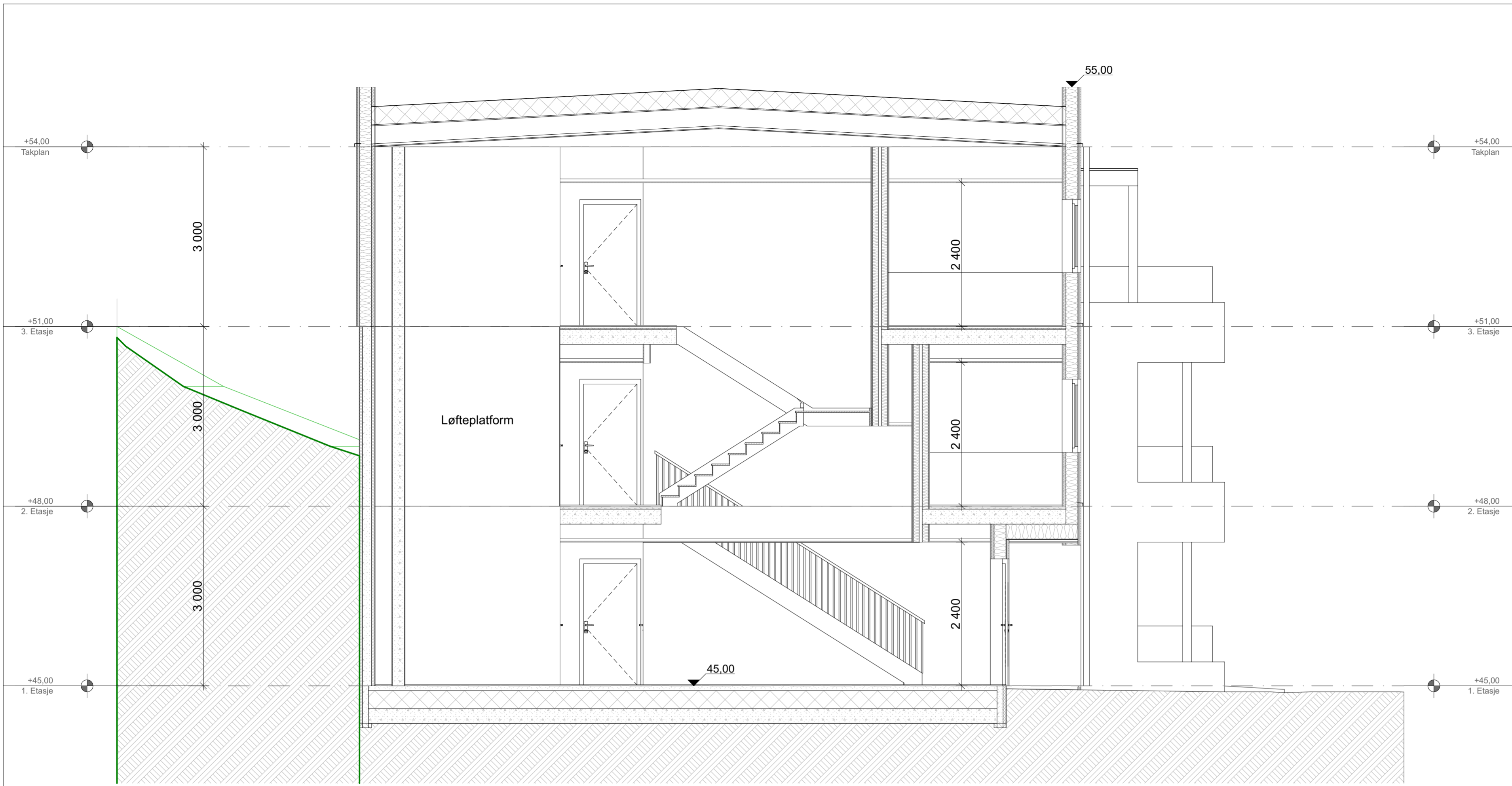
Snitt A-A
