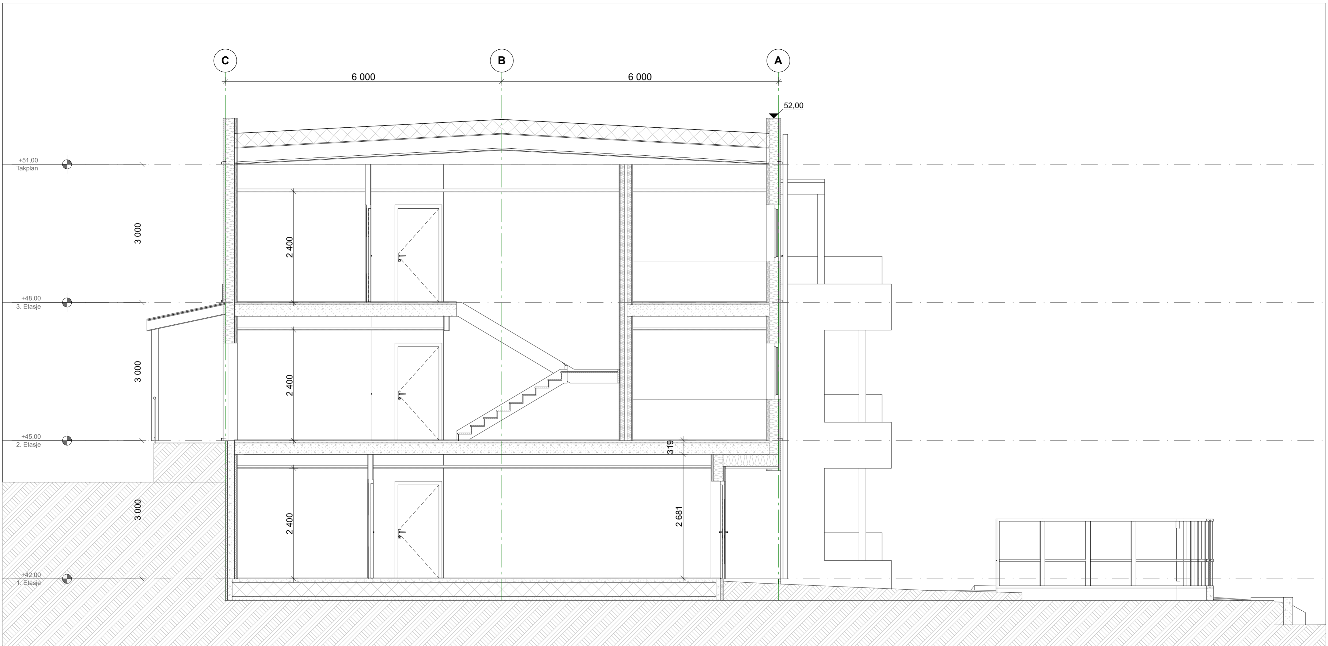
Snitt A-A
